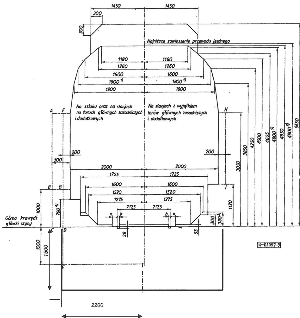
Rys. 3. Skrajnia budowli linii zelektryfikowanych z siecią górną dla nowych budowli ciężkich, tj. takich których stateczność umożliwia zakotwienie linki nośnej przewodów jezdnych trakcji elektrycznej (skrajnia C)
