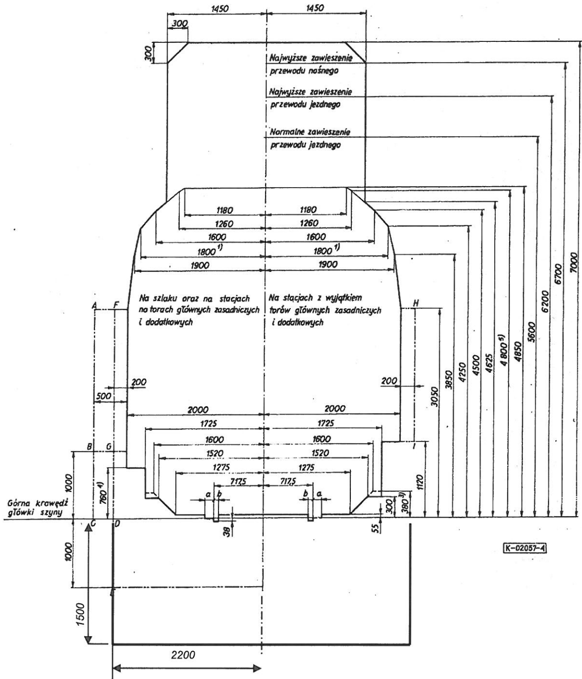
Rys. 4. Skrajnia budowy linii zelektryfikowanych z siecią górną dla nowych budowli lekkich tj. takich których stateczność uniemożliwia zakotwienie linki nośnej przewodów jezdnych trakcji elektrycznej (skrajnia D)
