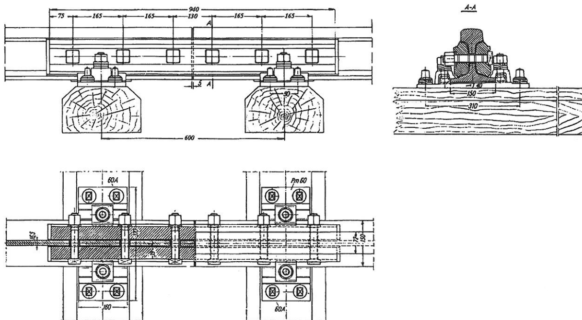
Rys. 1 Złącze szyn 60E1 wiszące
