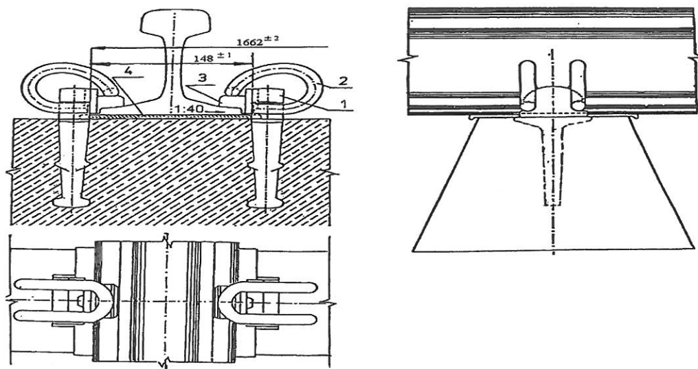
Rys. 2 Przytwierdzenie typu SB szyny 49E1 do podkładów betonowych Oznaczenia: 1- kotwa, 2- łapka sprężysta, 3- elektroizolacyjna wkładka dociskowa, 4- przekładka podszynowa.
