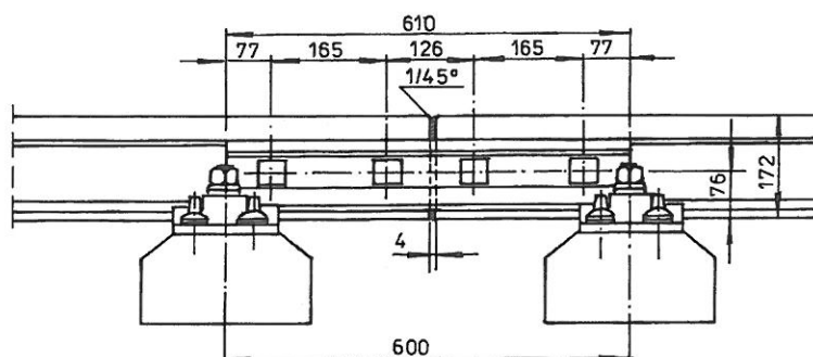
Rys. 3 Złącze szynowe izolowane klejono-sprężone z łóbkami czterootworowymi
