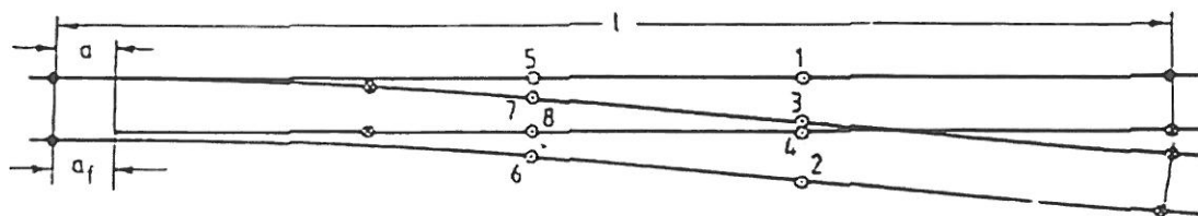
Rys. 3 Kolejność spawania rozjazdu
