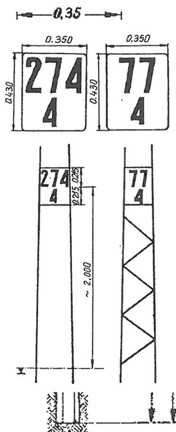
Rys. 1 Znaki kilometrowe i hektometrowe niskie na liniach niezelektryfikowanych Rys. 2 Znaki kilometrowe i hektometrowe wysokie na liniach niezelektryfikowanych
