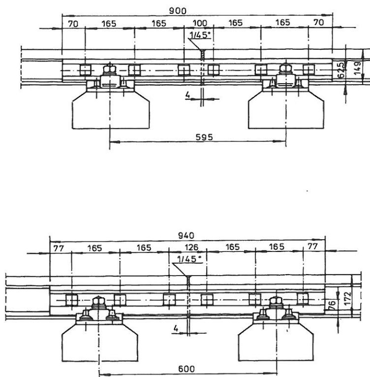
Rys. 2 Złącze szynowe izolowane klejono-sprężone z łóbkami sześciotworowymi Rysunek górny: szyny 49E1, rysunek dolny szyny 60E1
