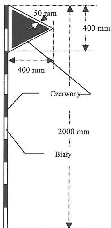
Rys. 8.1 Wskaźnik oznaczający kierunek zejścia z toru
