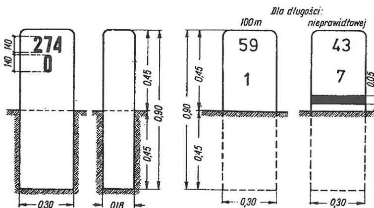
Rys. 1 Znaki kilometrowe i hektometrowe niskie na liniach niezelektryfikowanych Rys. 2 Znaki kilometrowe i hektometrowe wysokie na liniach niezelektryfikowanych
