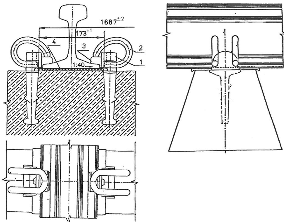
Rys.1 Przytwierdzenie typu SB szyny 60E1 do podkładów betonowych Oznaczenia: 1- kotwa, 2- łapka sprężysta, 3- elektroizolacyjna wkładka dociskowa, 4- przekładka podszynowa.
