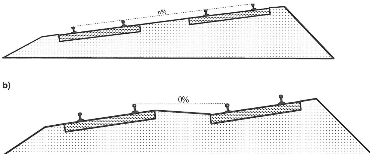
Rys 3.2. Kształtowanie przejazdu na torze w łuku a. Wszystkie toki szynowe wzdłuż linii prostej (na jednakowym pochyleniu n\% ) b. Wewnętrzne toki szynowe obu torów na jednym poziomie
