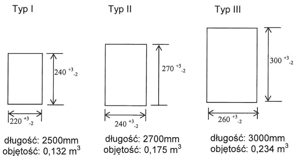
Rys. 3 Typy mostownic
