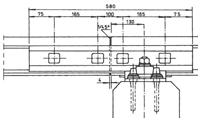
Rys. 4 Złącze szynowe izolowane klejono-sprężone z łóbkami czterootworowymi
